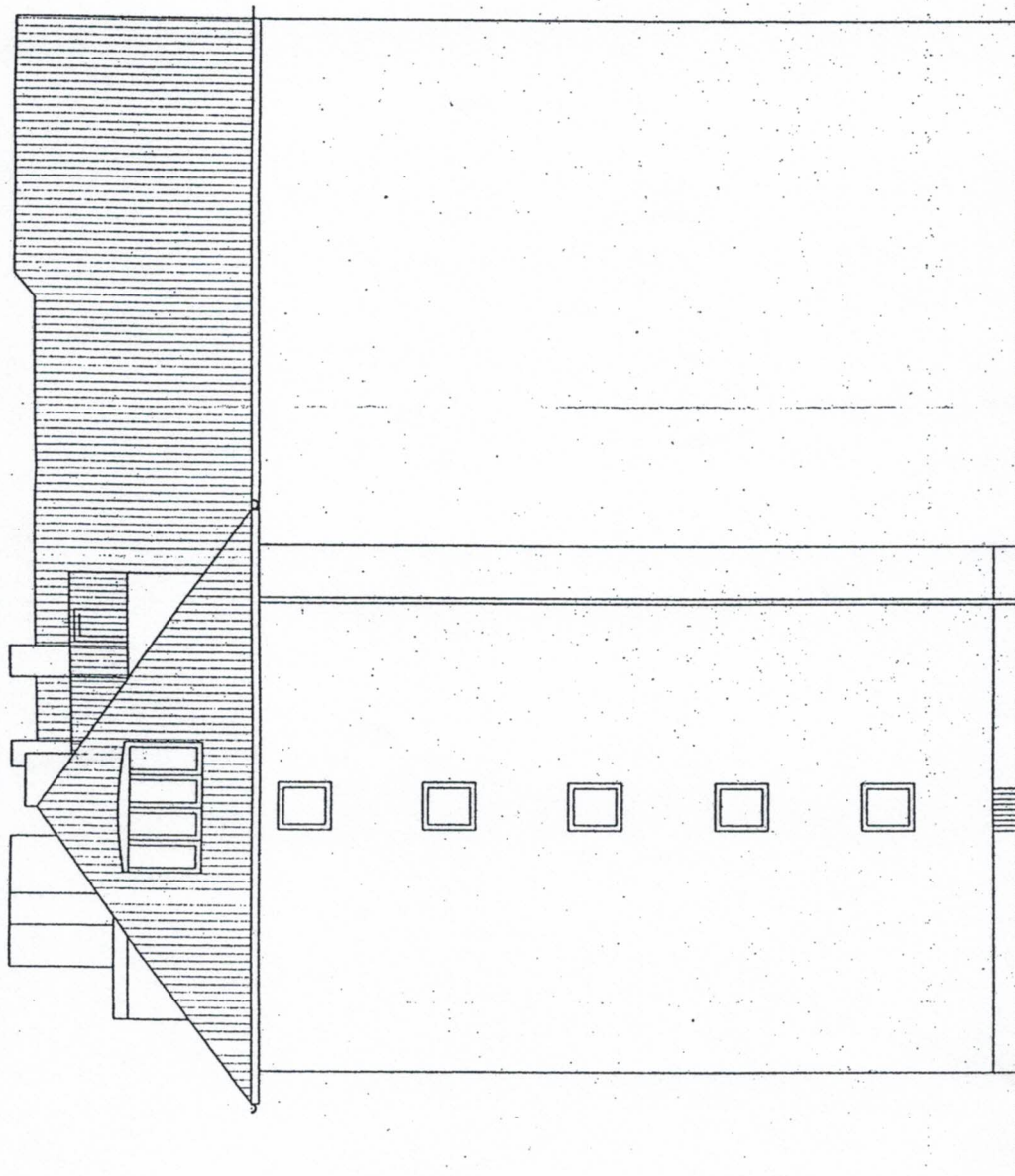
ANSICHT WEST
